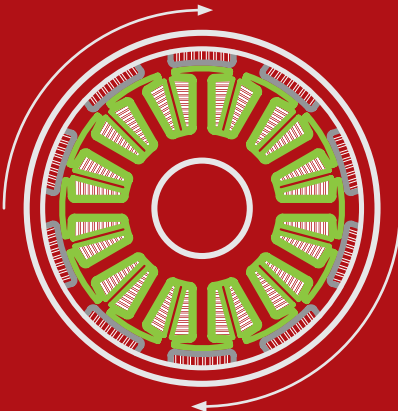
Außenrotor-Motor
