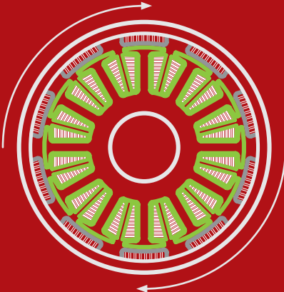
Außenrotor-Motor
