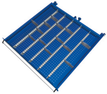
Modell SGB-B04-...(Bestellzusatz BZ)
