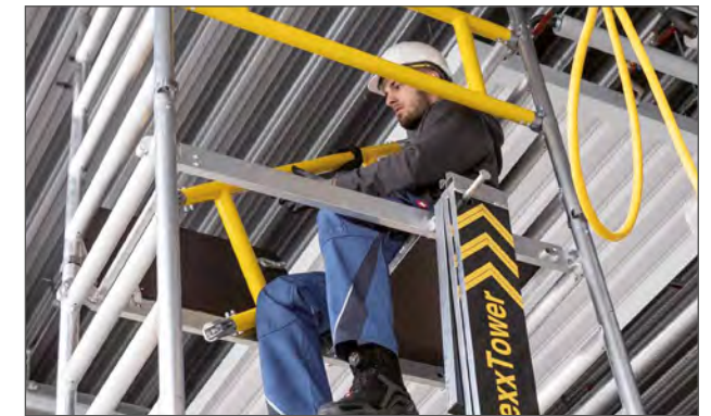
Obere Geländer und Bordbretter montieren
