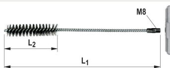
Reinigungsbürste BS
